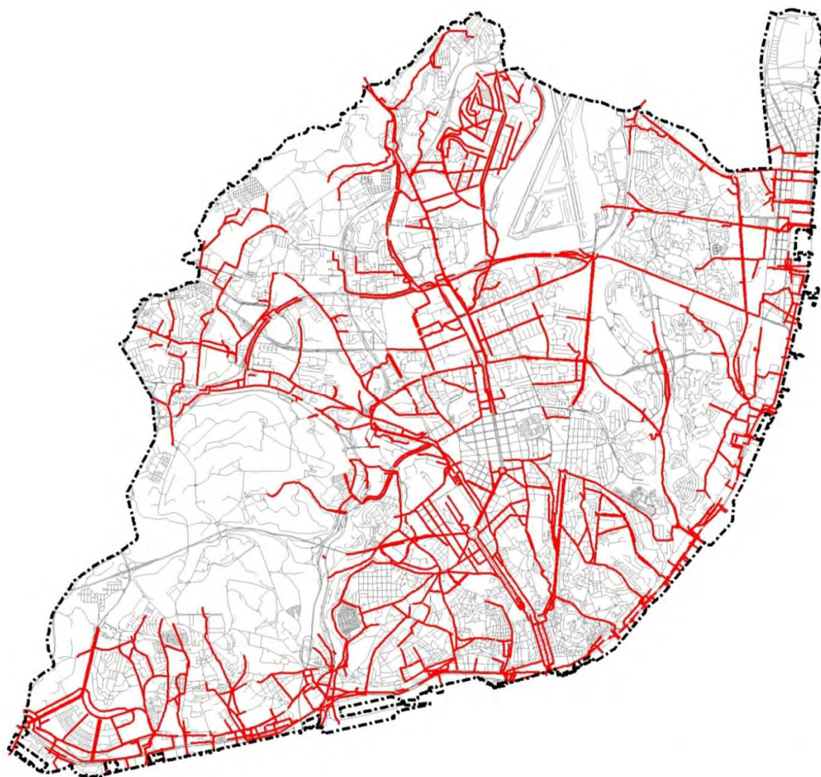
Figura 8.2 - Rede principal do sistema de drenagem
