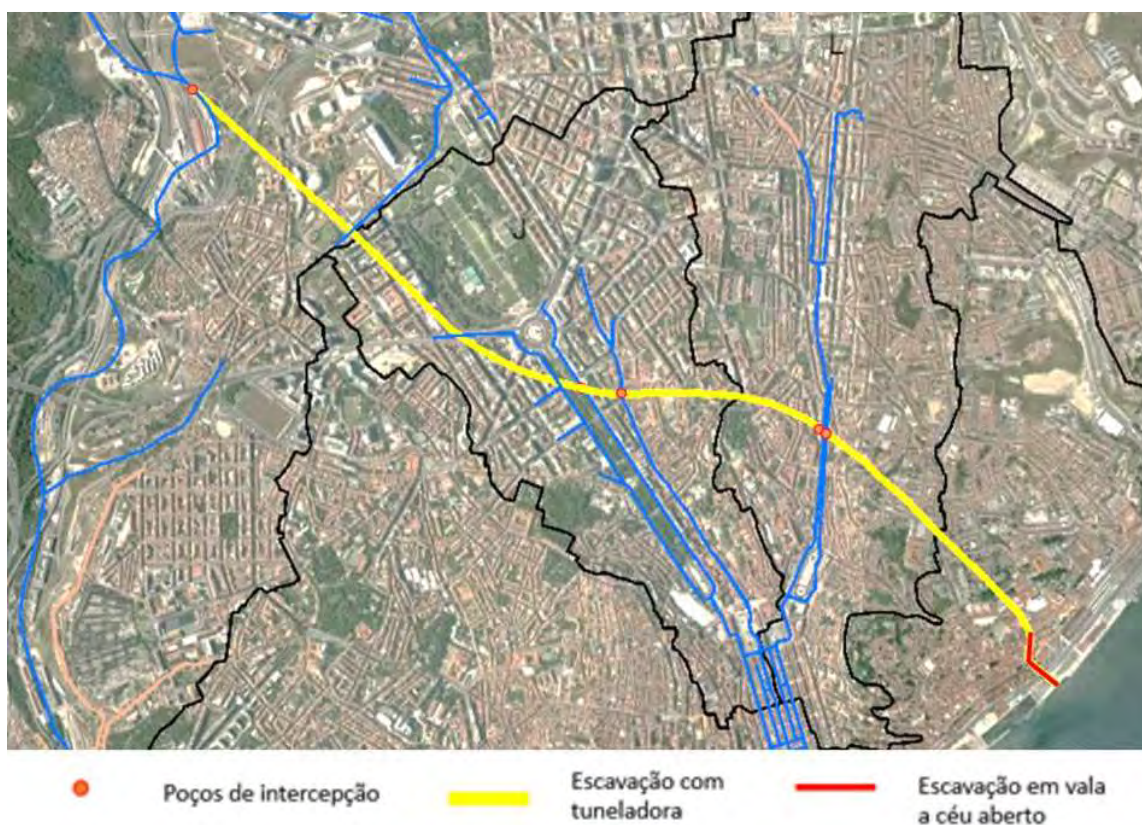
Figura 8.4 – Traçado do Túnel de drenagem Monsanto - Stª Marta - Stª Apolónia
