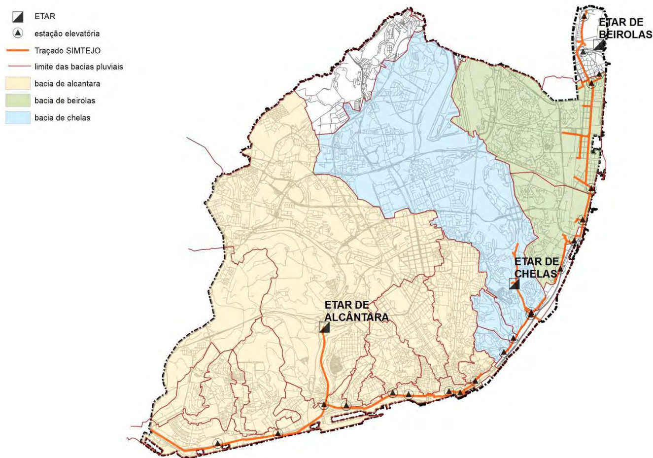
Figura 8.3 – Áreas abrangidas pelas estações de tratamento da cidade de Lisboa
