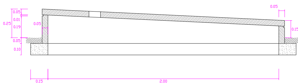
Corte BB'
