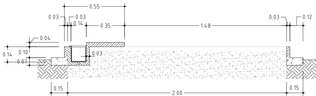
CORTE AB
