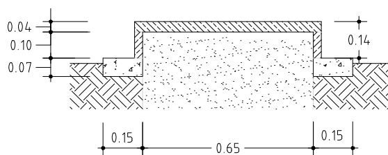
CORTE CD
