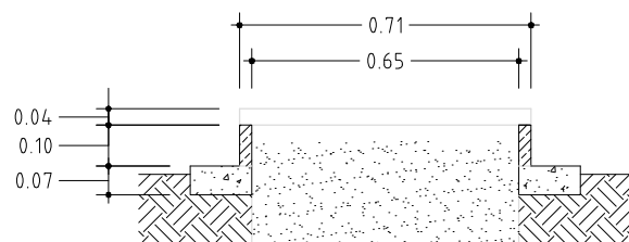
CORTE AB
