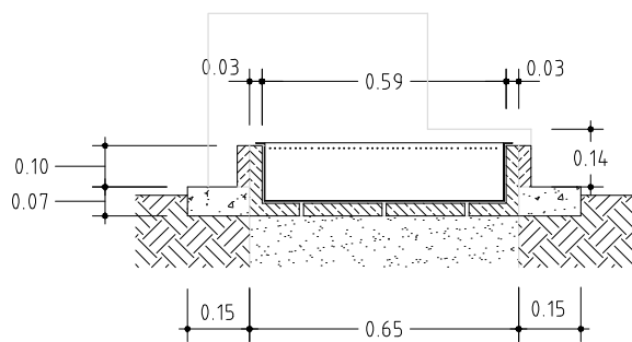
CORTE GH
