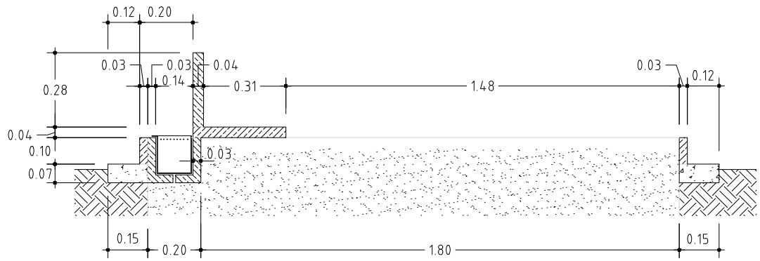
CORTE AB
