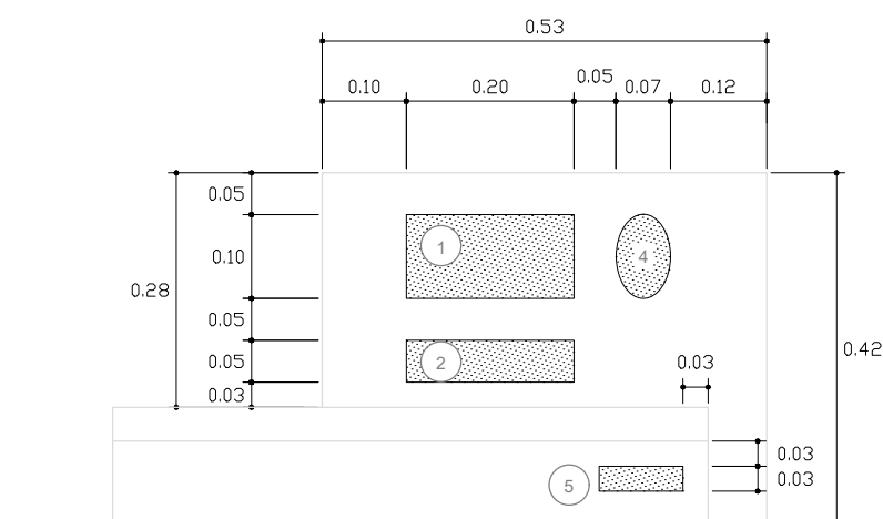
ALÇADO ANTERIOR
