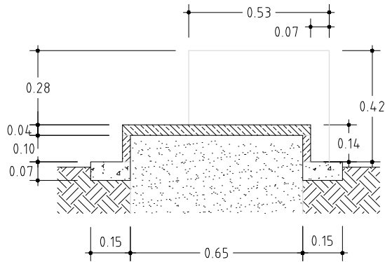
CORTE CD
