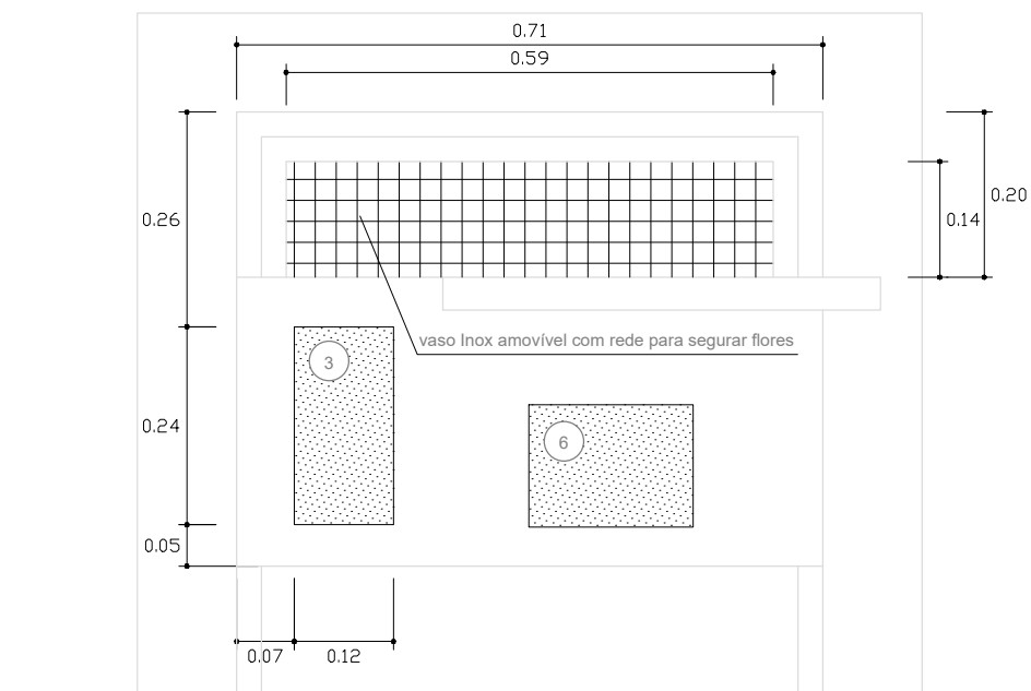
PLANTA
